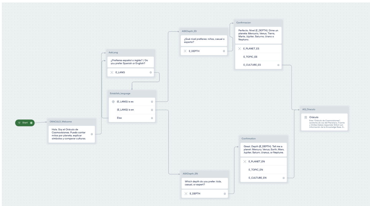
Figura 1: Diagrama de Bloques en VoiceFlow
