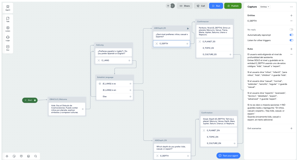
Figura 3: Obtención del nivel de profundidad solicitado por el usuario (análogo en inglés)
