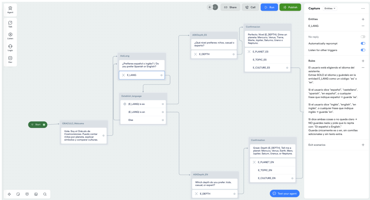
Figura 2: Obtención del idioma solicitado por el usuario
