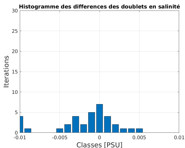
Figure 9 : Répartition du nombre des écarts de salinité
