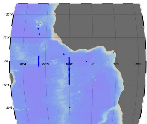
Figure 2 : Carte des stations hydrographiques (profils CTD) de la mission PIRATA FR35
