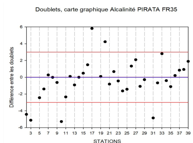
Figure 23 : Carte graphique des doublets pour la mesure de l'alcalinité totale (en fonction des stations), mission PIRATA FR35
