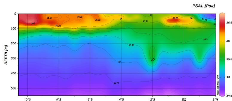
Figure 5 : Représentation graphique des mesures de la salinité réalisées sur la radiale 10W, PIRATA FR35
