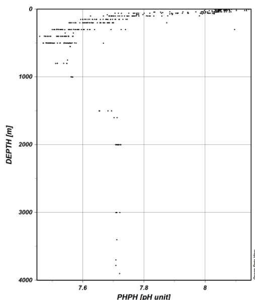
Figure 16 : Représentation graphique des mesures de pHt (@25) sur l'ensemble des profils PIRATA FR35
