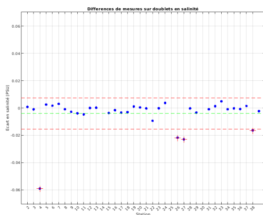
Figure 7 : Ecart des doublets des mesures de la salinité au cours de la mission PIRATA FR35
