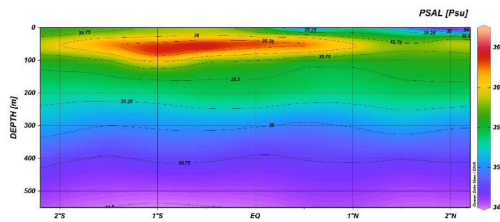
Figure 6 : Représentation graphique des mesures de la salinité réalisées sur la radiale 23W, PIRATA FR35
