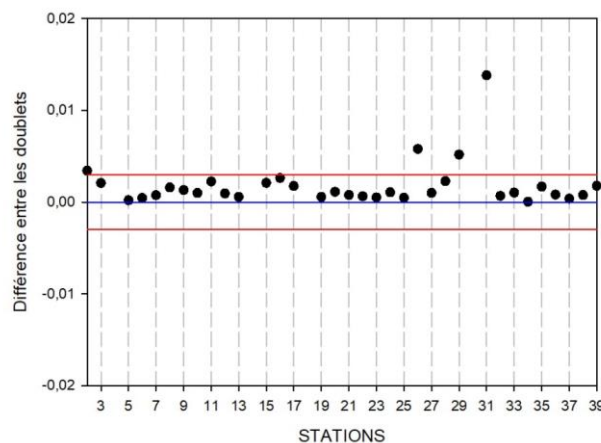
Figure 19 : Carte graphique des doublets pour la mesure du pH t (en fonction des stations), mission PIRATA FR35
