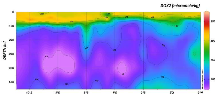
Figure 11 : Représentation graphique des mesures de l'oxygène dissous réalisées sur la radiale 10W, PIRATA FR35
