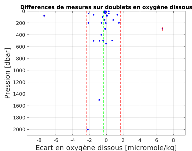
Figure 14 : Ecart des doublets des mesures de l'oxygène dissous en fonction de la profondeur de prélèvement
