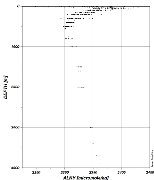
Figure 20 : Représentation graphique des mesures d'alcalinité totale sur l'ensemble des profils PIRATA FR35
