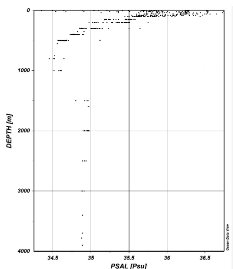
Figure 3 : Représentation graphique des mesures de salinité sur l'ensemble des profils PIRATA FR35
