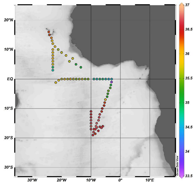
Figure 4 : Représentation graphique des mesures de salinité sur l'ensemble des prélèvements de surface PIRATA FR35
