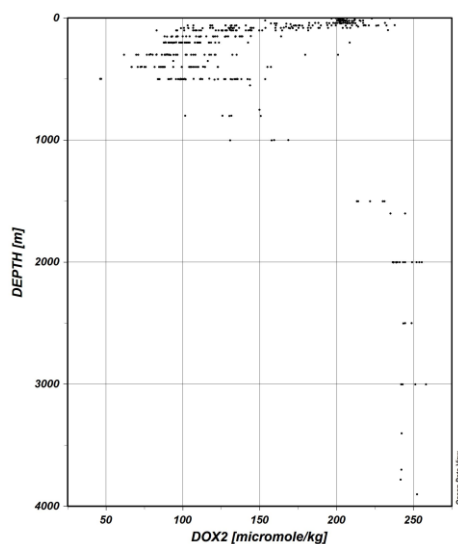
Figure 10 : Représentation graphique des mesures de l'oxygène dissous sur l'ensemble des profils PIRATA FR35
