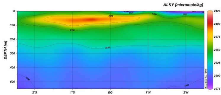
Figure 22 : section 10 W, alcalinité totale, PIRATA FR35
