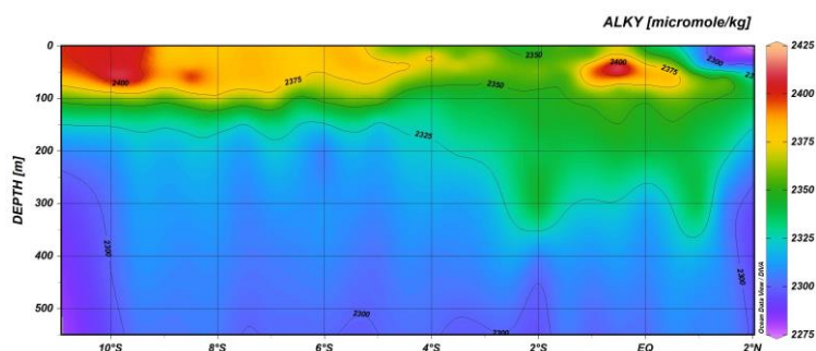
Figure 21 : section 10 W, alcalinité totale, PIRATA FR35
