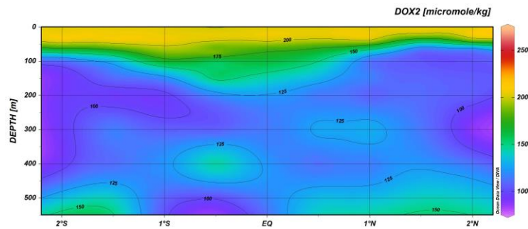
Figure 12 : Représentation graphique des mesures de l'oxygène dissous réalisées sur la radiale 23W, PIRATA FR35
