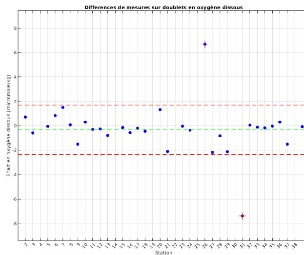
Figure 13 : Ecart des doublets des mesures de l'oxygène dissous au cours des stations
