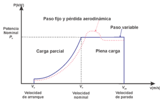
Figura 5: Curva típica de potencia de un aerogenerador
