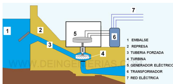
Figura 6: Esquema básico de una central hidroeléctrica
