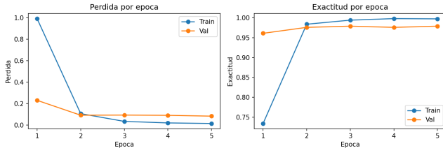
Fig. 1. Curvas de pérdida (izquierda) y exactitud (derecha) por época sobre los conjuntos de entrenamiento y validación. Generadas desde el notebook de entrenamiento.
