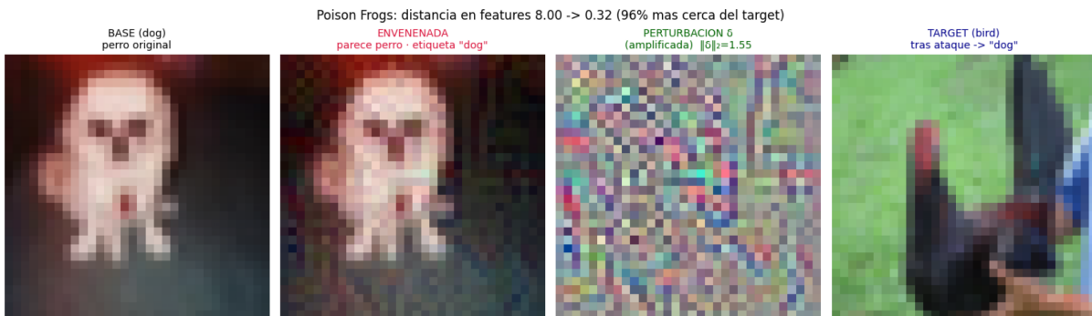
Figura 6: Ataque clean-label (Poison Frogs) en transfer-learning. De izquierda a derecha: imagen base (un perro real, etiqueta dog ); imagen envenenada (visualmente sigue siendo un perro y conserva la etiqueta dog , pero sus features colisionan con el objetivo); la perturbación \delta amplificada (de magnitud pequeña, \ell_2 = 1.55 ); y el objetivo (un pájaro que, tras inyectar el veneno en el fine-tuning , se clasifica como dog ). La distancia en el espacio de features entre base y objetivo se reduce un 96% ( 8.00 \rightarrow 0.32 ): la imagen parece un perro pero la red la procesa casi como el pájaro.
