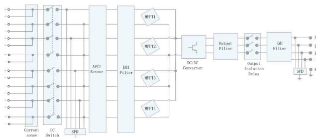
Diagrama del circuito
