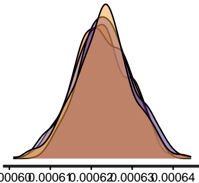
phi2
