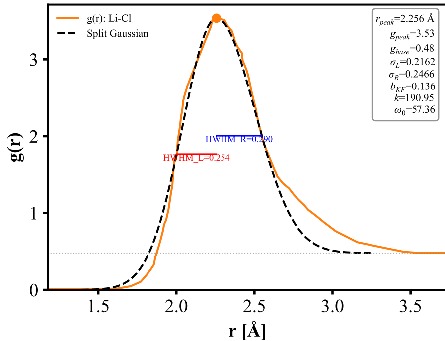
Li-Cl
