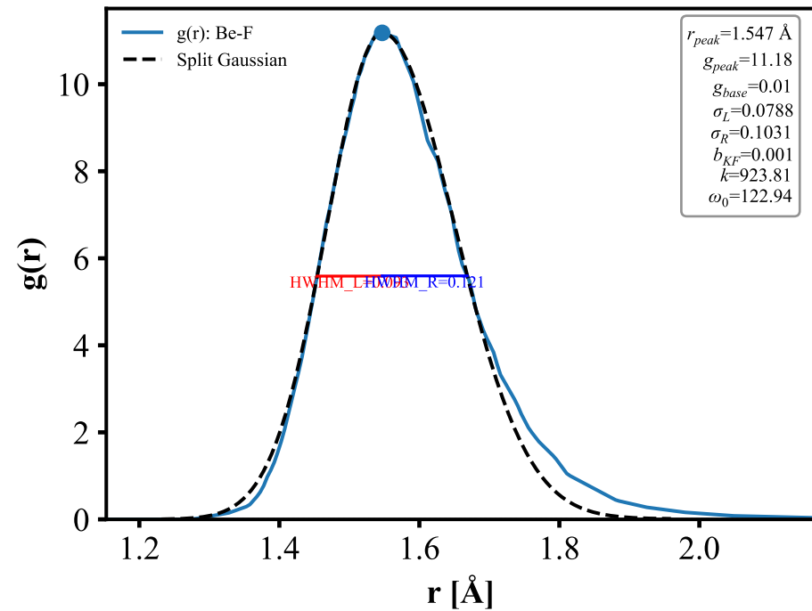
Be-F
