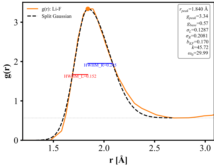
Li-F
