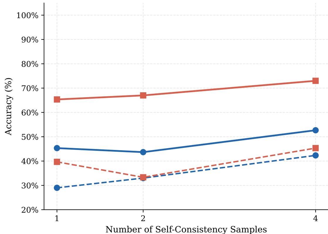
SVAMP
