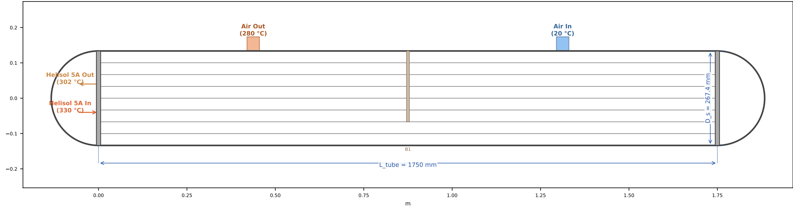
Sheet 2 - Longitudinal Section
