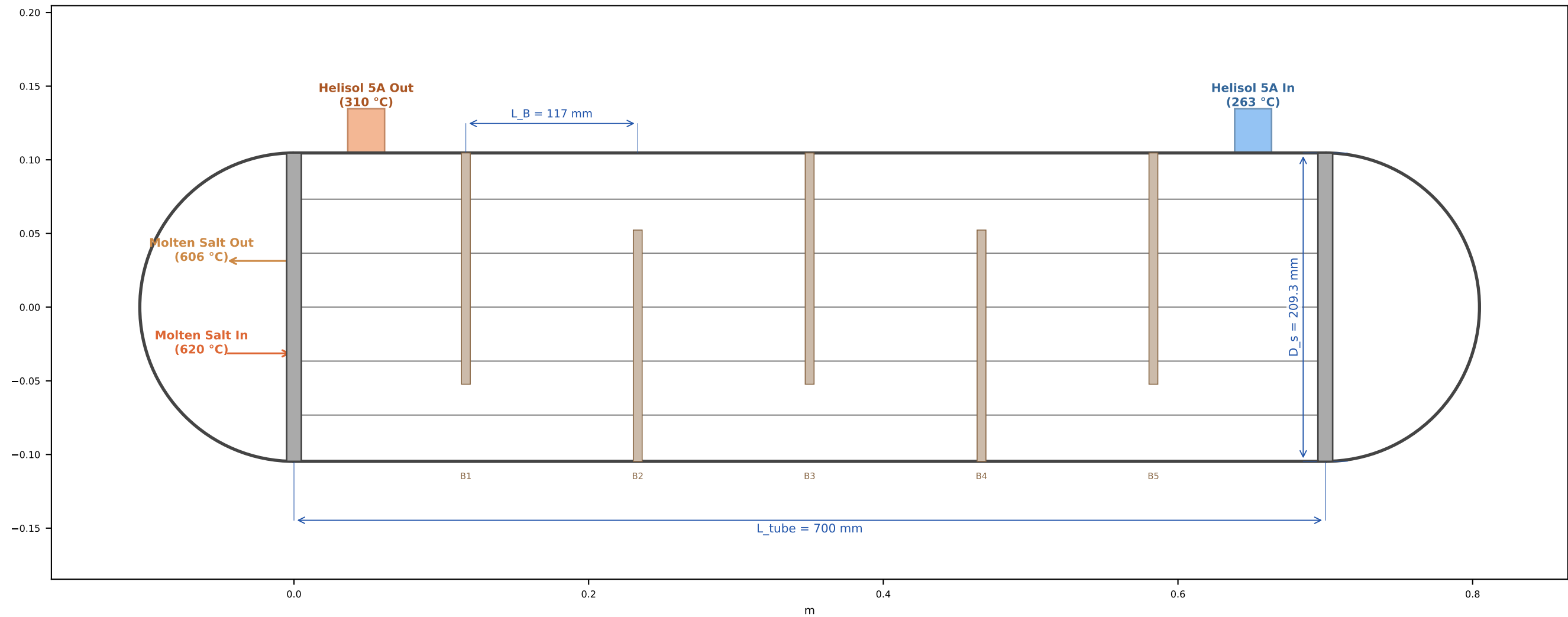
Sheet 2 - Longitudinal Section
