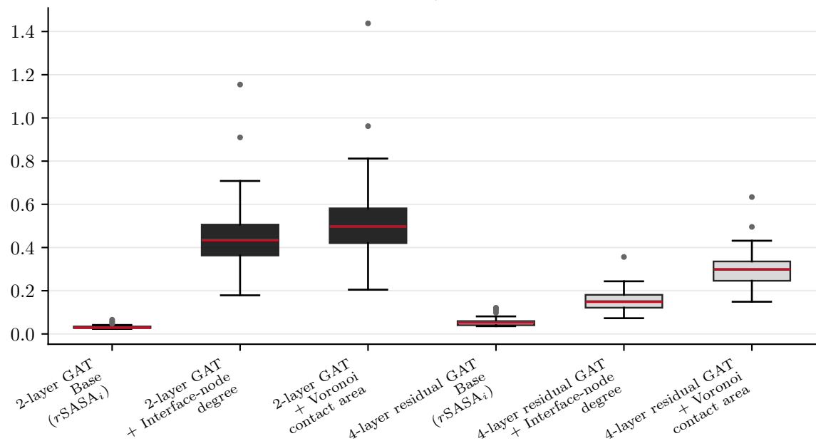
rSASA_i MAE
