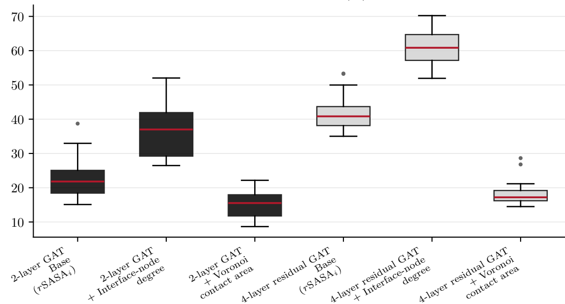
Interface-edge F1 (%)
