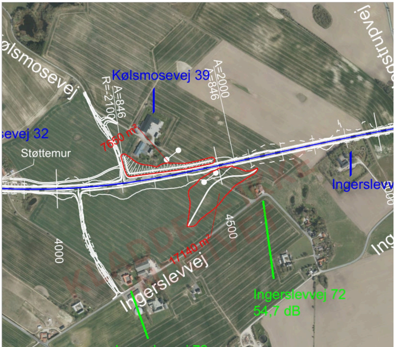
B4, Kølslosevej/Ingerslevvej — udsnit af bilag 61. Screeningsafgørelsen angår volden syd for vejen, som efter afgørelsen dækker 17.200 m 2 . Kortet påtegner arealet syd for vejen 17140 m 2 . Det røde areal nord for vejen (7650 m 2 ) er et andet anlæg.
