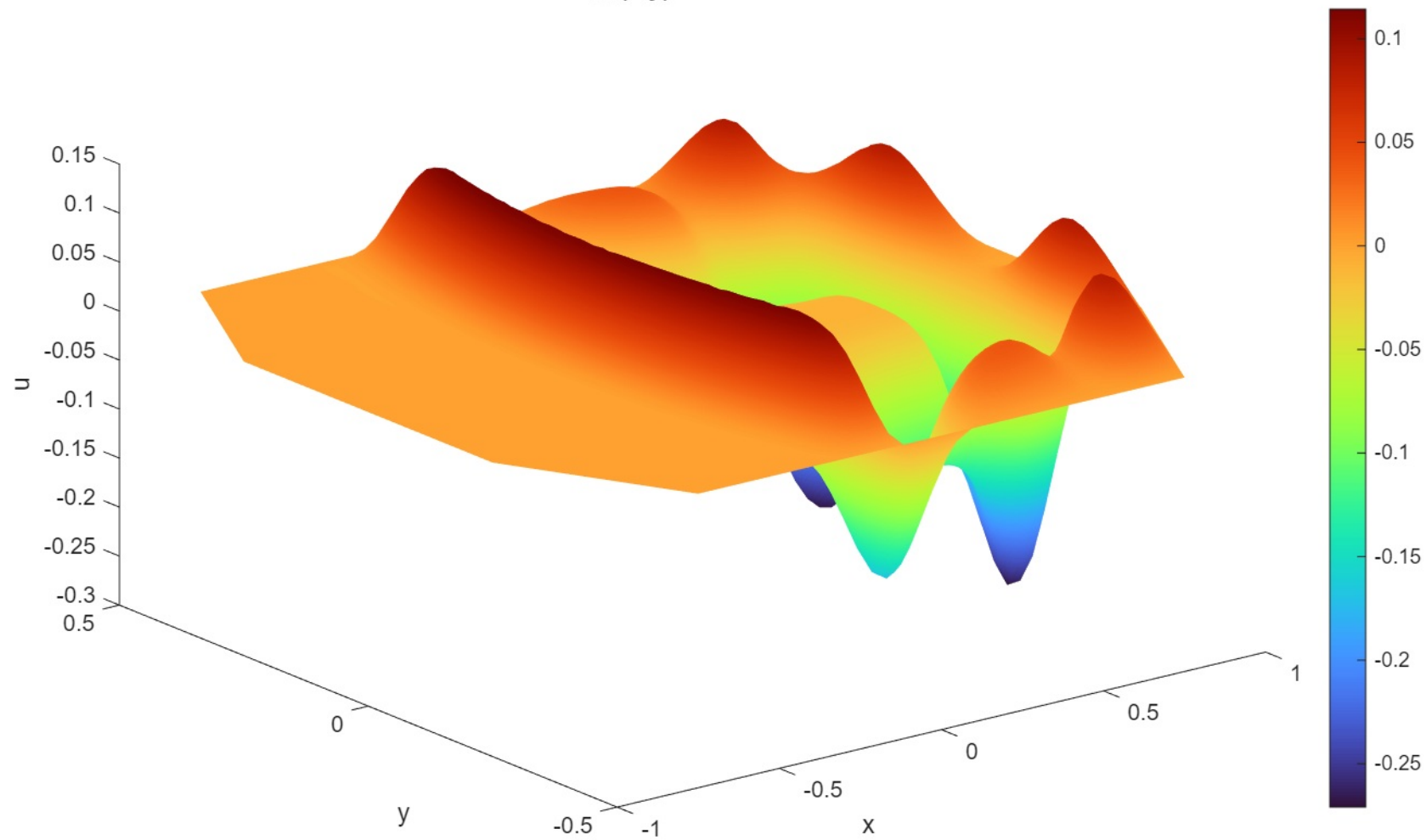
u_{2.5}(x,y) - Dirichlet
