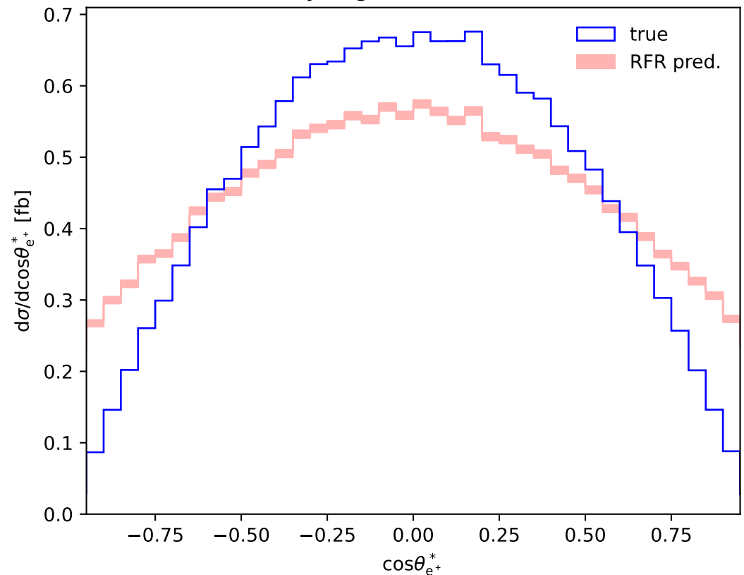
Positron decay angle (NLO QCD, LHE, fiducial)
