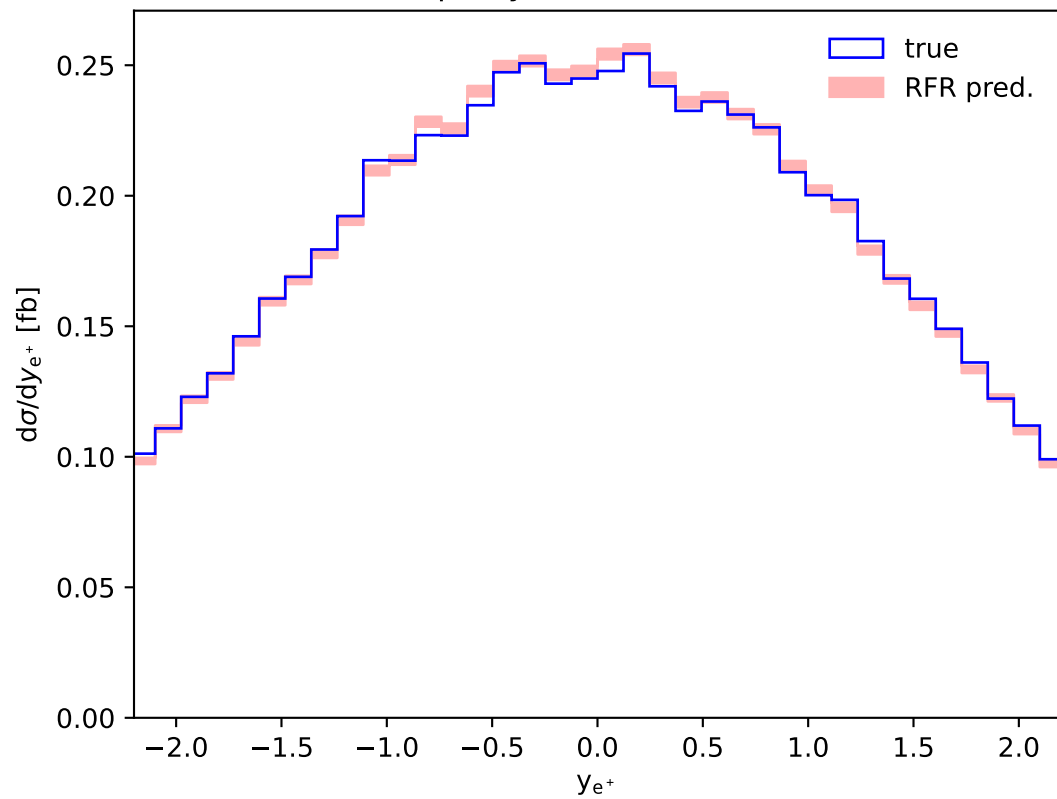
Positron rapidity (NLO QCD, LHE, fiducial)
