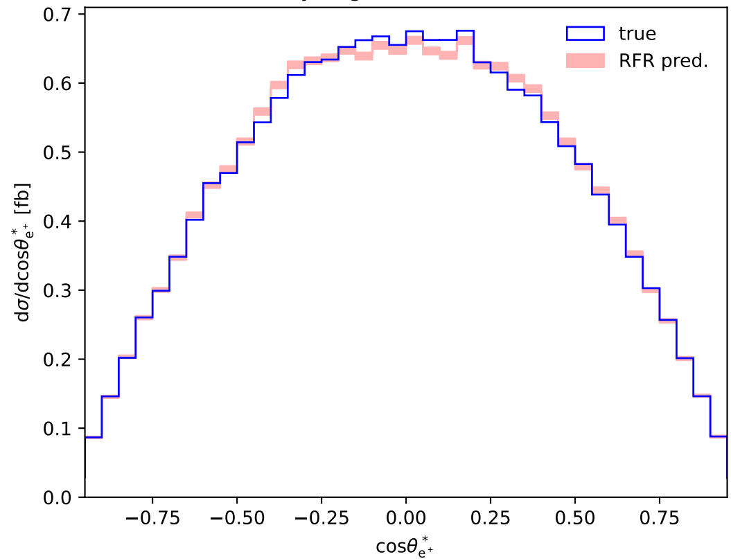
Positron decay angle (NLO QCD, LHE, fiducial)
