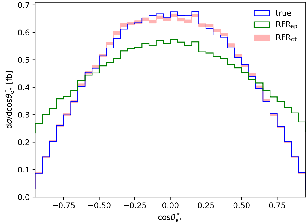
Positron decay angle (NLO QCD, LHE, fiducial)
