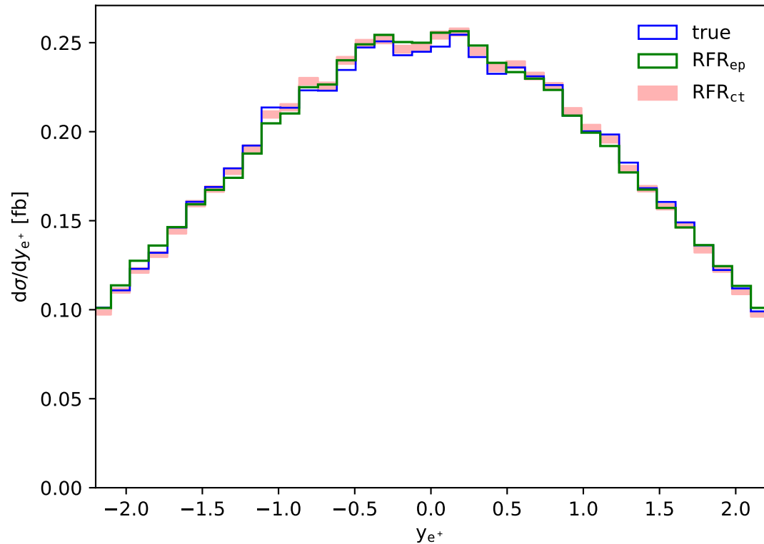
Positron rapidity (NLO QCD, LHE, fiducial)
