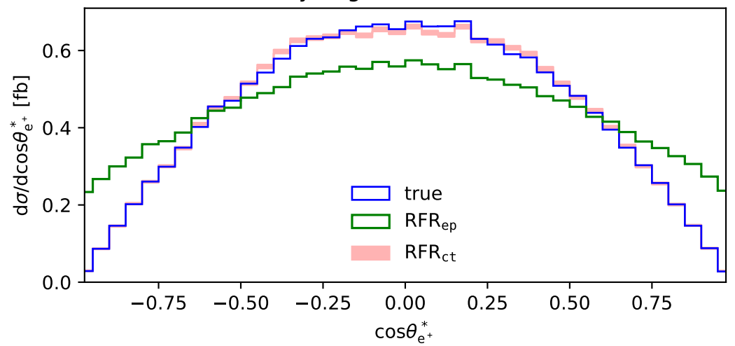
Positron decay angle (NLO QCD, LHE, fiducial)
