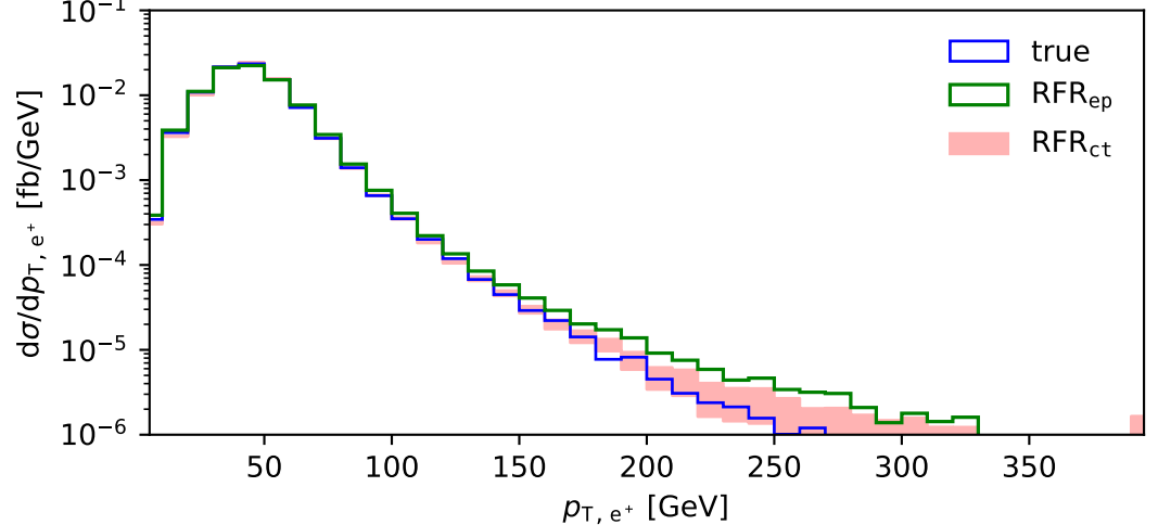
Positron transverse momentum (NLO QCD, LHE, fiducial)
