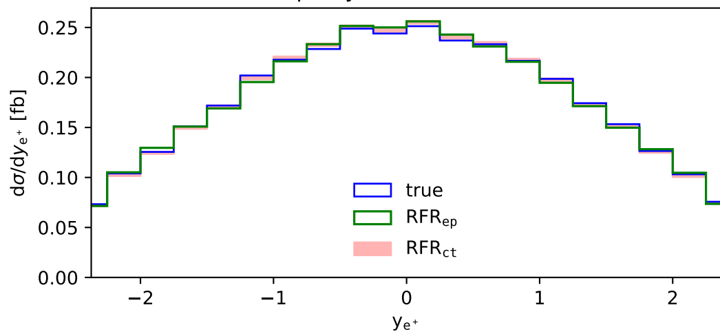
Positron rapidity (NLO QCD, LHE, fiducial)
