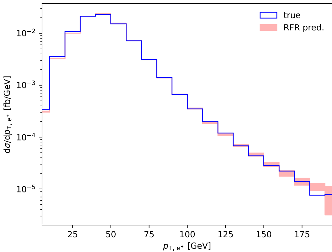
Positron transverse momentum (NLO QCD, LHE, fiducial)
