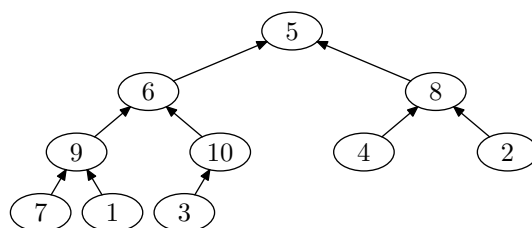
(d) After max-heapify on 3rd node.
