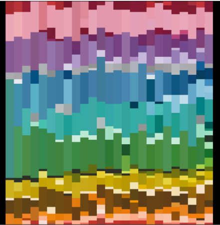
GPT-4
