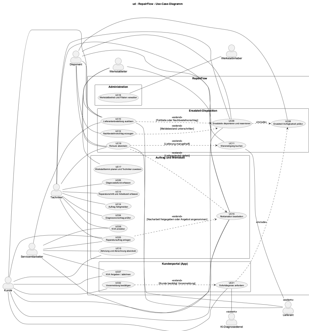
Abbildung 3: Use-Case-Diagramm RepairFlow
