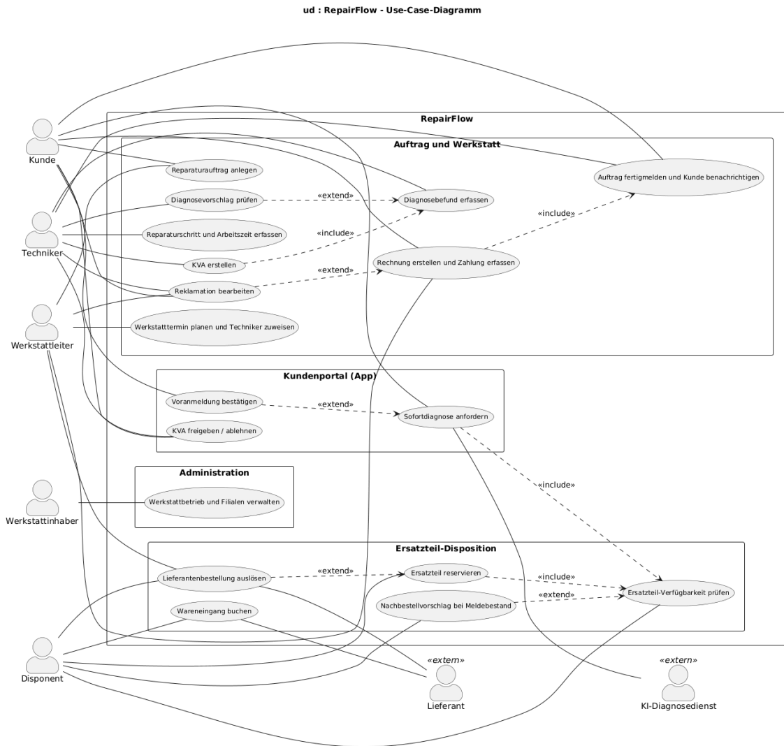
Abbildung 3: Use-Case-Diagramm RepairFlow
