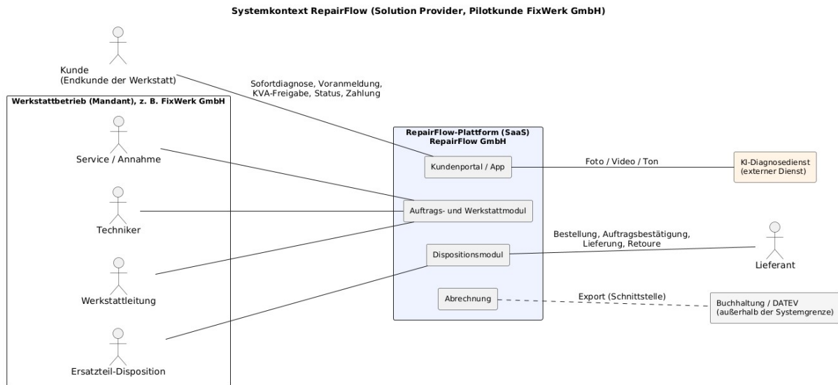
Abbildung 1: Systemkontext der RepairFlow-Plattform
