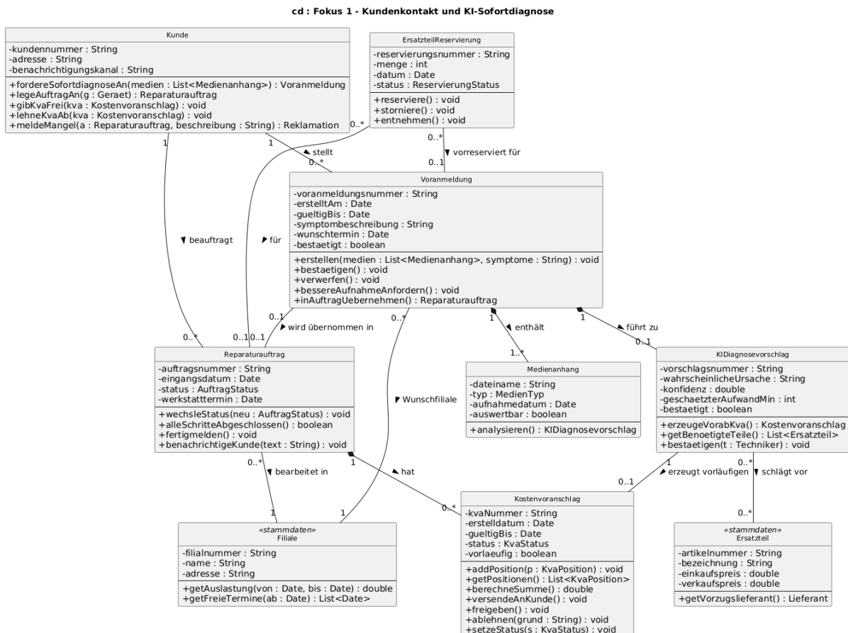
Abbildung 4: Klassendiagramm, Ausschnitt Kundenkontakt und KI-Sofortdiagnose
