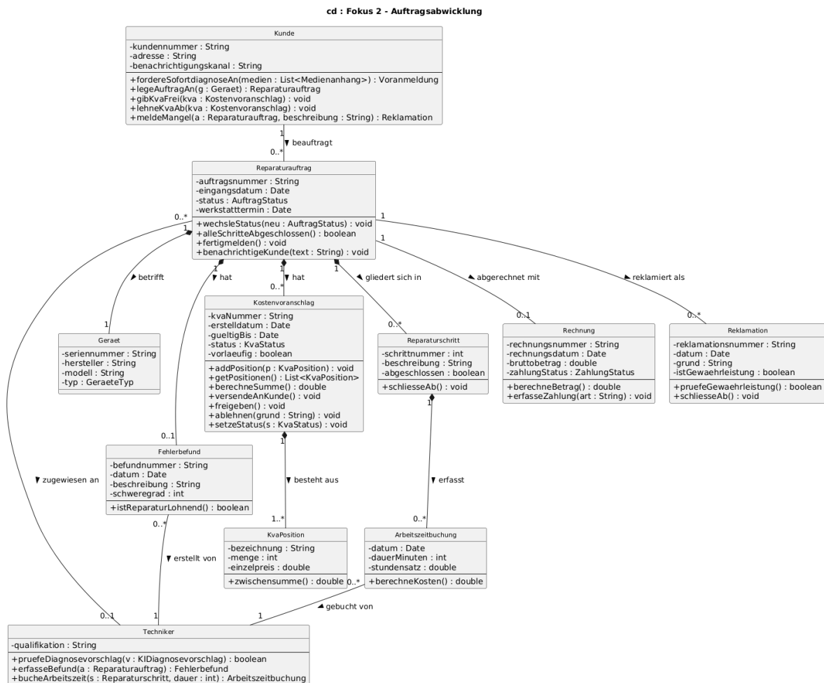
Abbildung 5: Klassendiagramm, Ausschnitt Auftragsabwicklung
