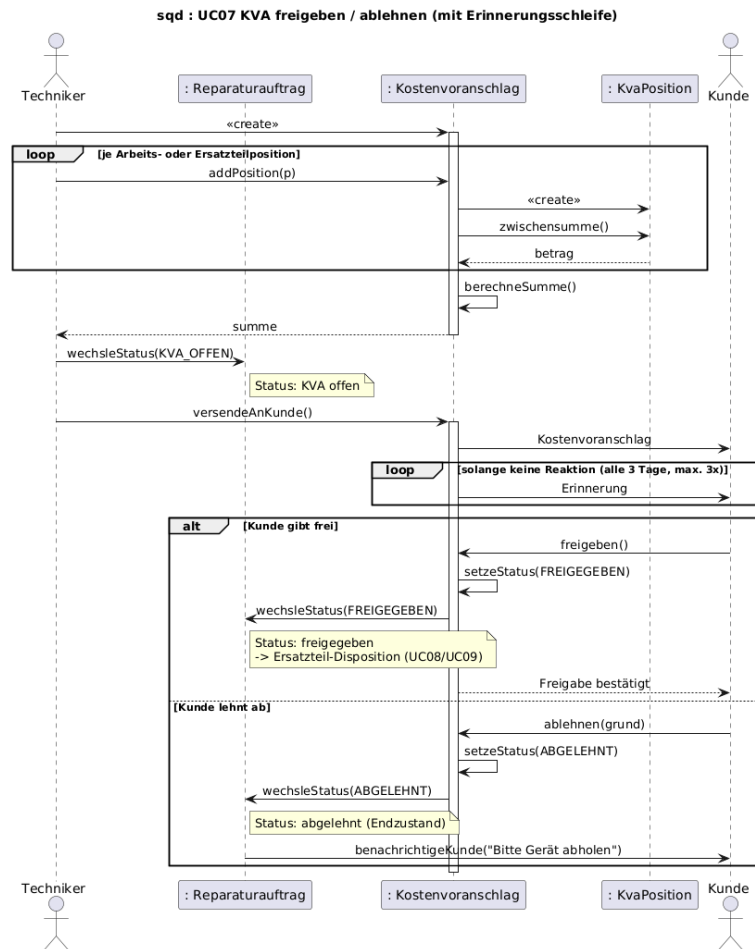
Abbildung 7: SD2 – KVA freigeben / ablehnen (UC07)
