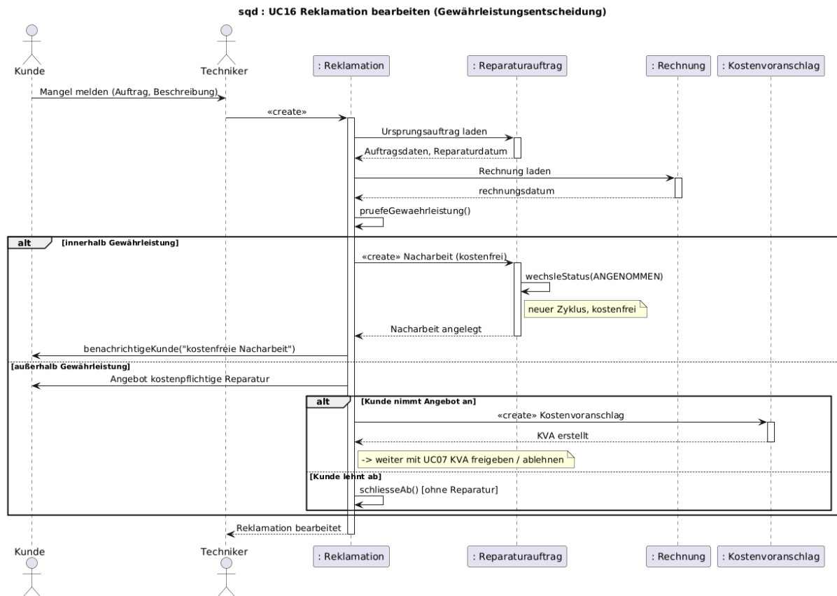
Abbildung 10: SD5 – Reklamation bearbeiten (UC16)
