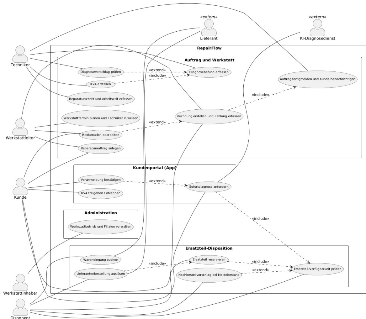
Abbildung 3: Use-Case-Diagramm RepairFlow
