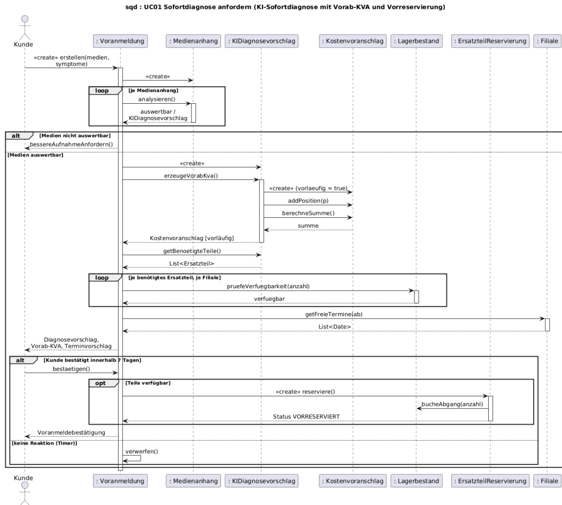
Abbildung 6: SD1 – Sofortdiagnose anfordern (UC01)
