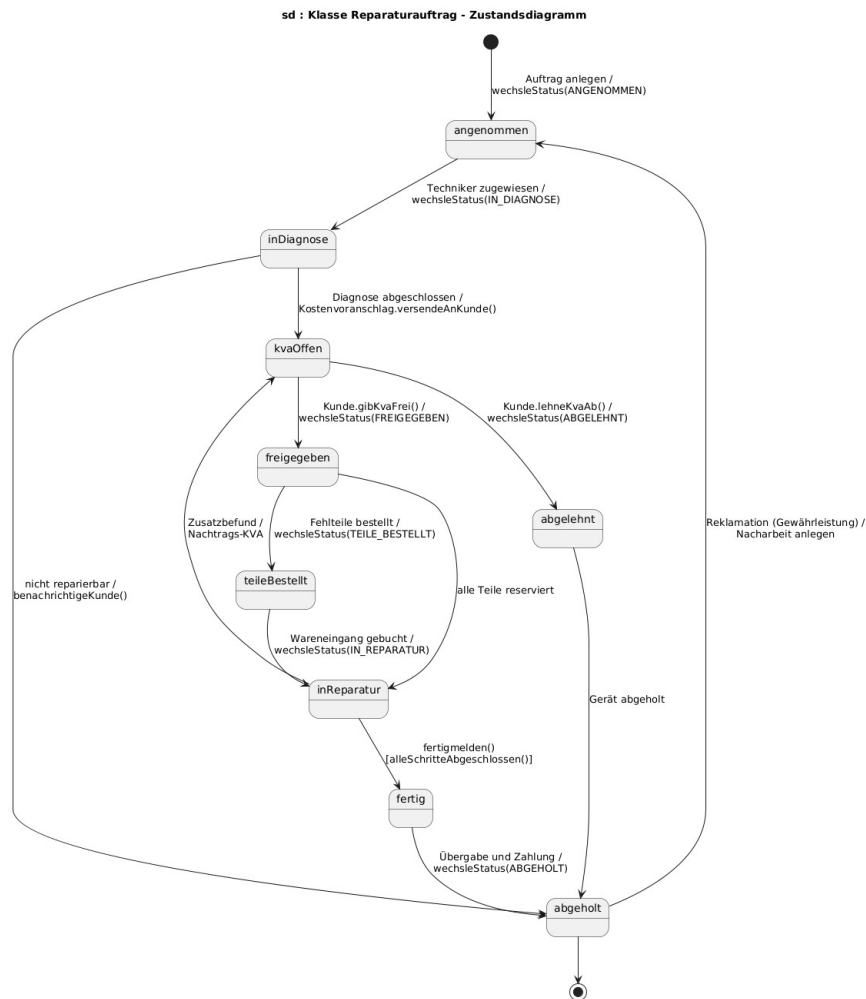
Abbildung 2: Zustandsdiagramm der Klasse Reparaturauftrag
