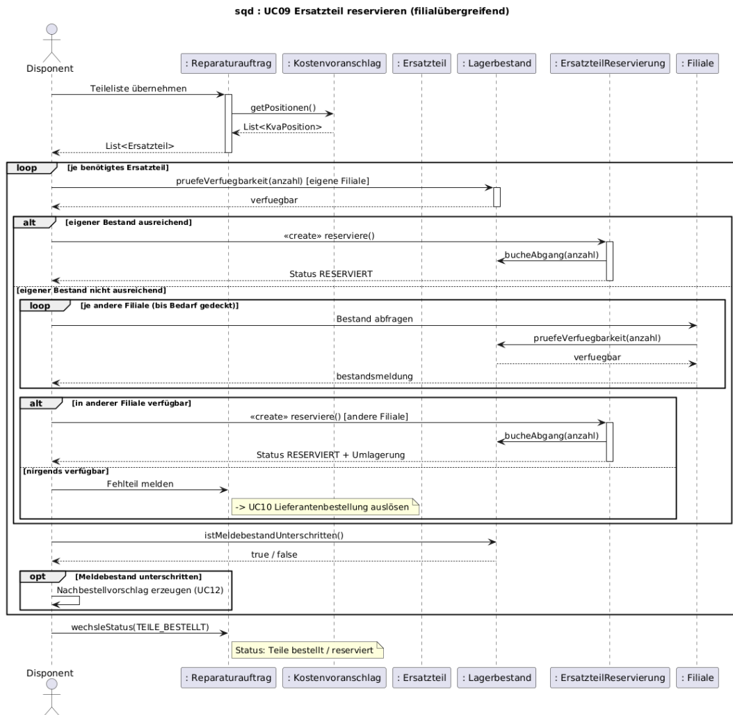
Abbildung 8: SD3 – Ersatzteil reservieren, filialübergreifend (UC09)
