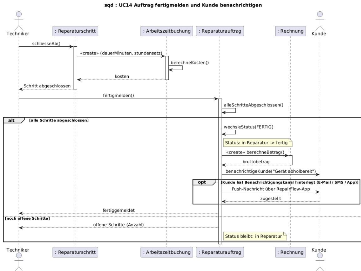
Abbildung 9: SD4 – Auftrag fertigmelden und Kunde benachrichtigen (UC14)
