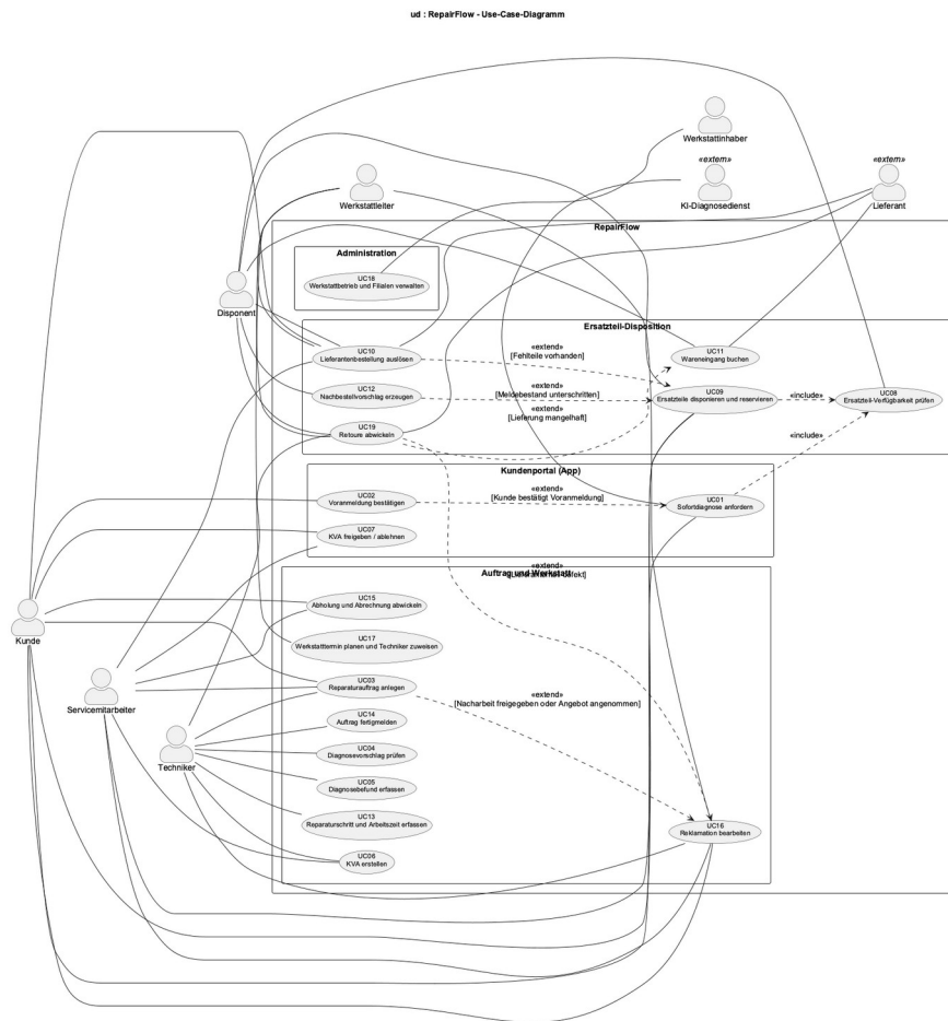
Abbildung 3: Use-Case-Diagramm RepairFlow
