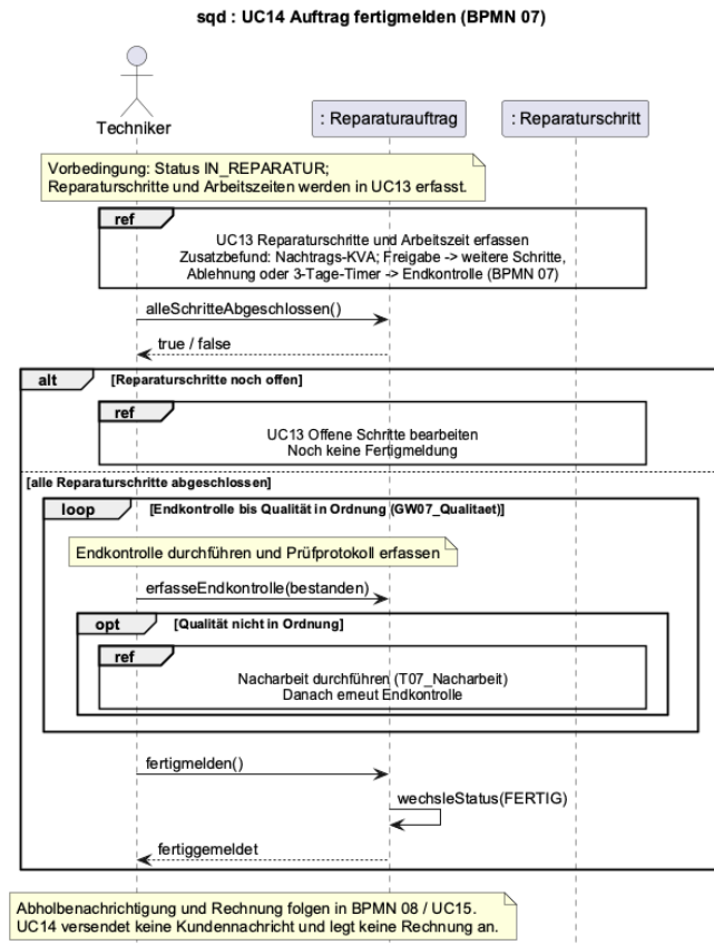
Abbildung 7: SD4 – Auftrag fertigmelden (UC14)
