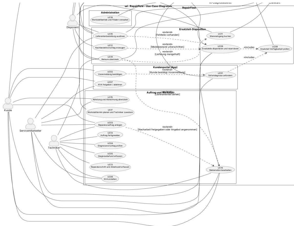
Abbildung 3: Use-Case-Diagramm RepairFlow
