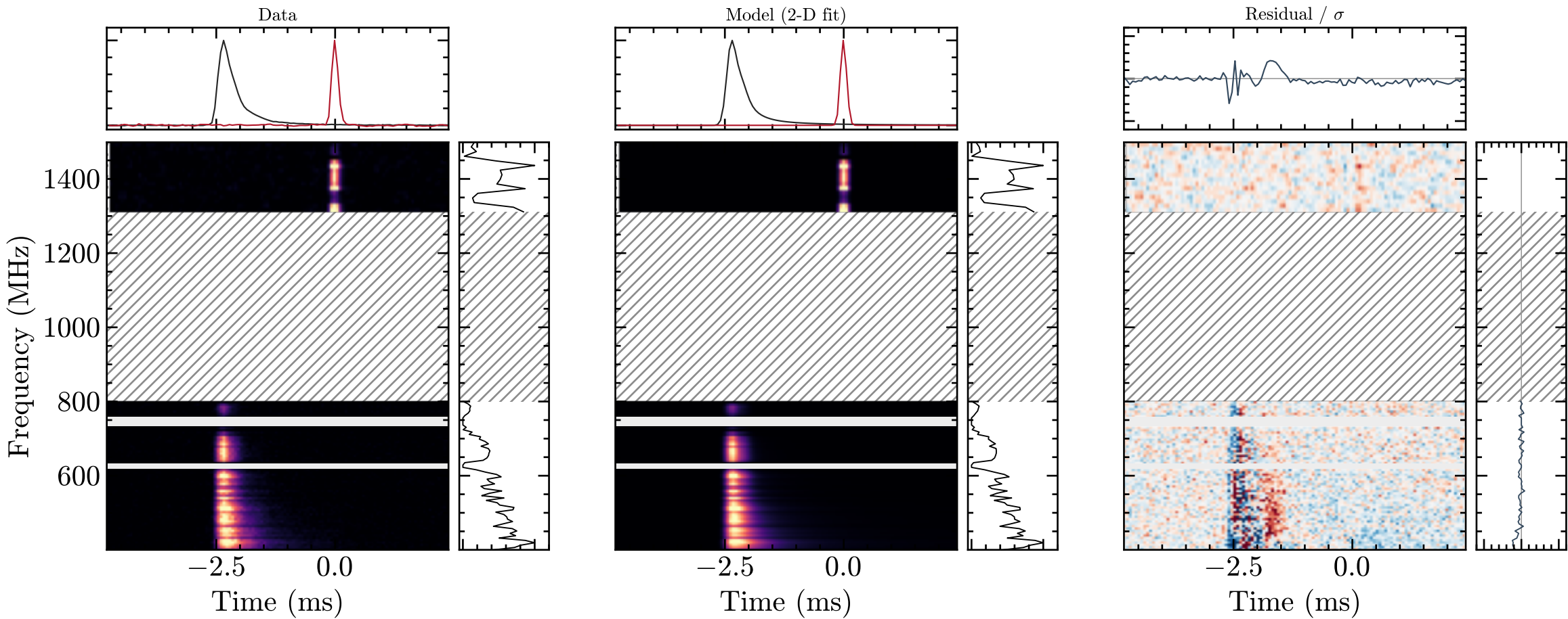
FRB 20240229A
