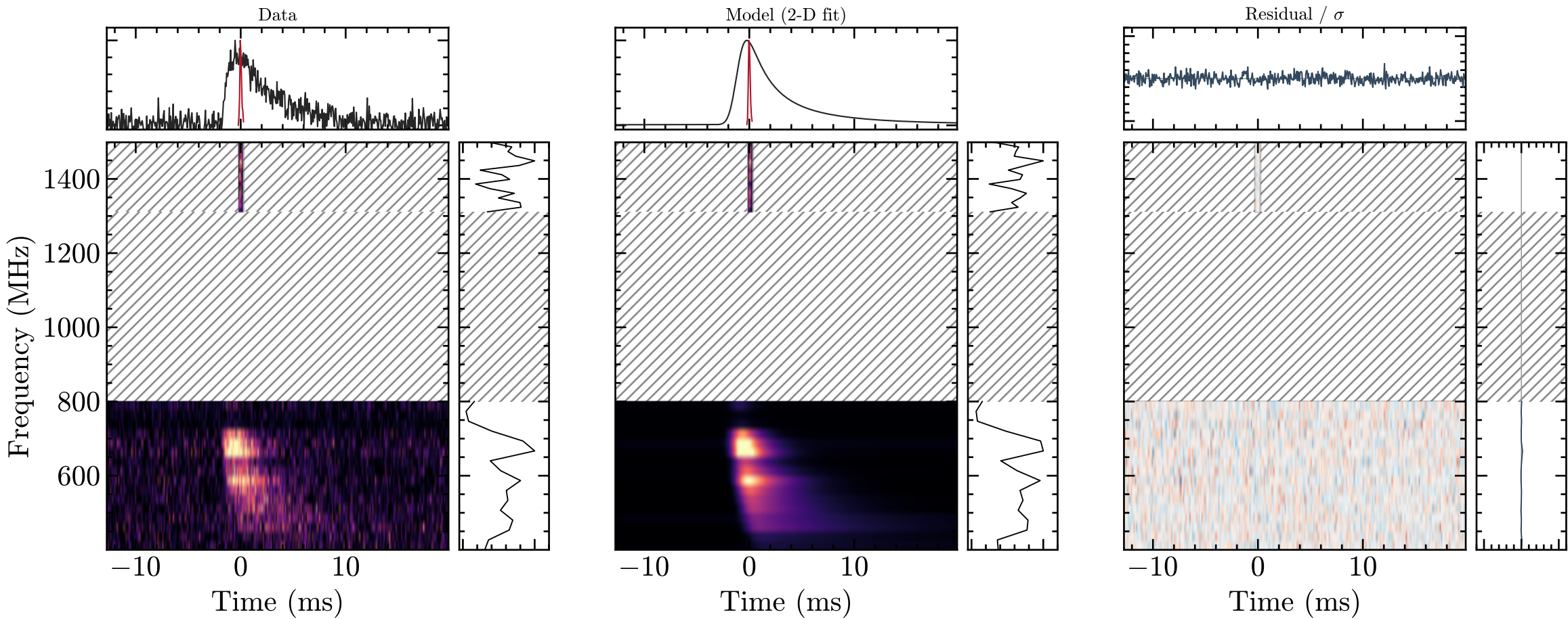
FRB 20221113A
