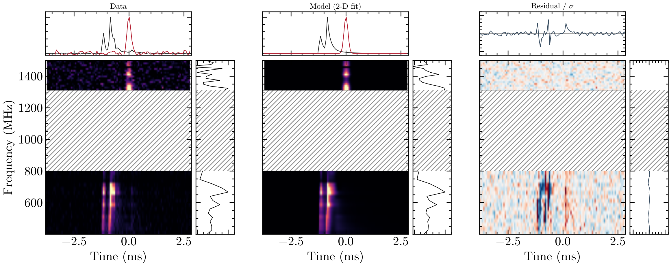
FRB 20230913A †
