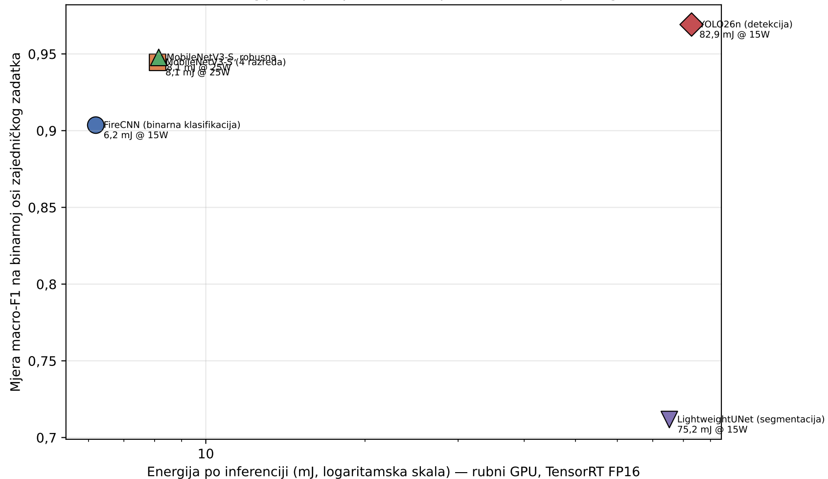
Točnost i energija: cijena po obrađenoj slici za svaku paradigmu
