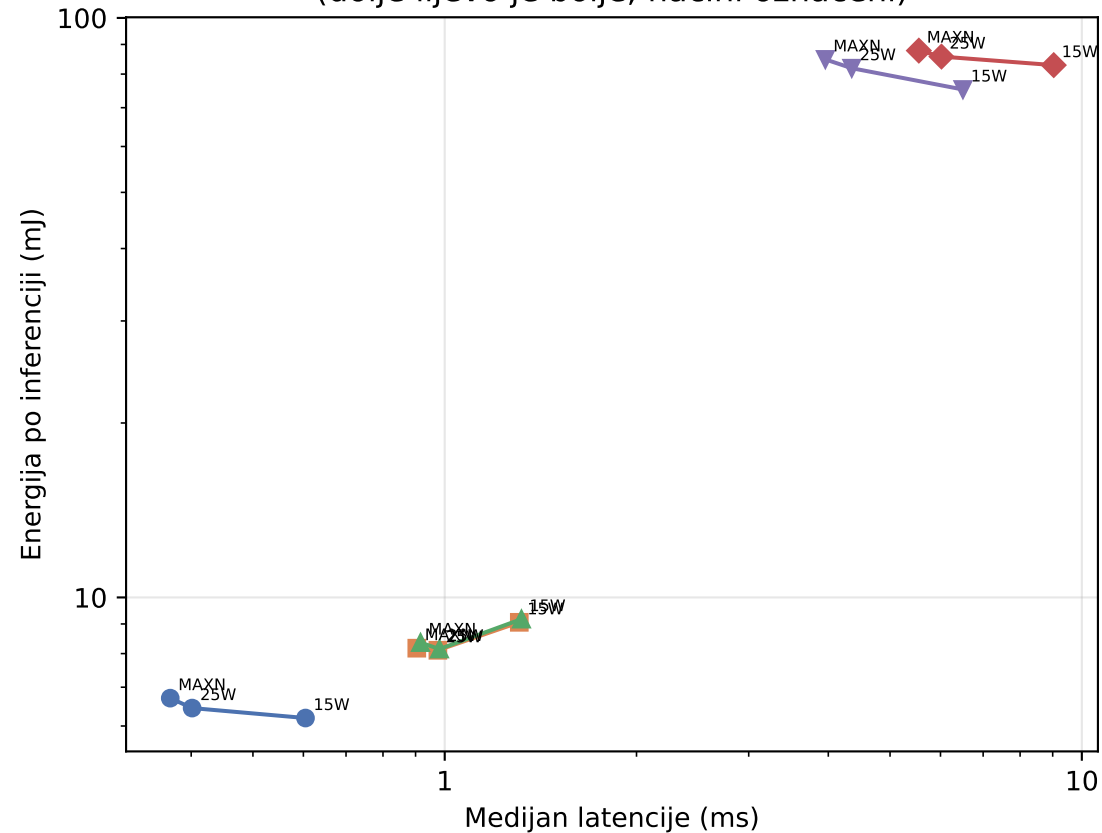
Odnos latencije i energije (dolje lijevo je bolje; načini označeni)
