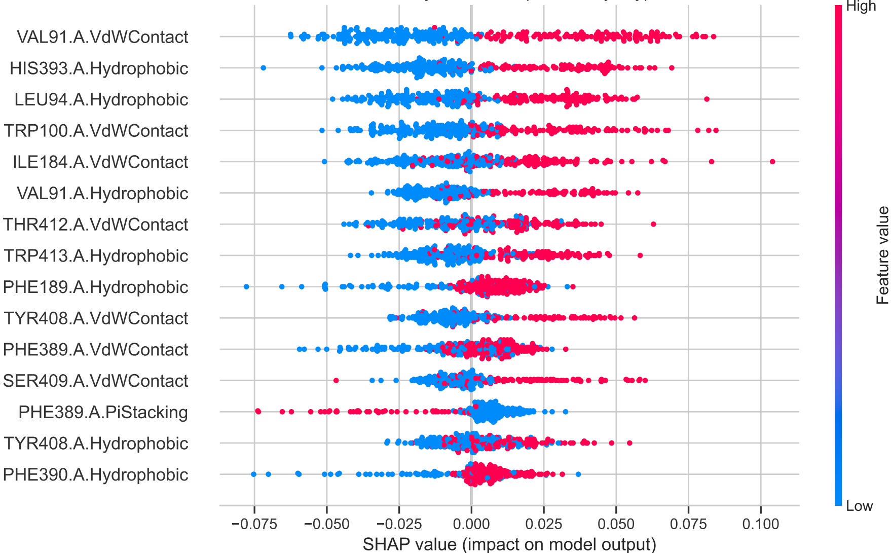
D2 – wykres SHAP (klasa: aktywny)
