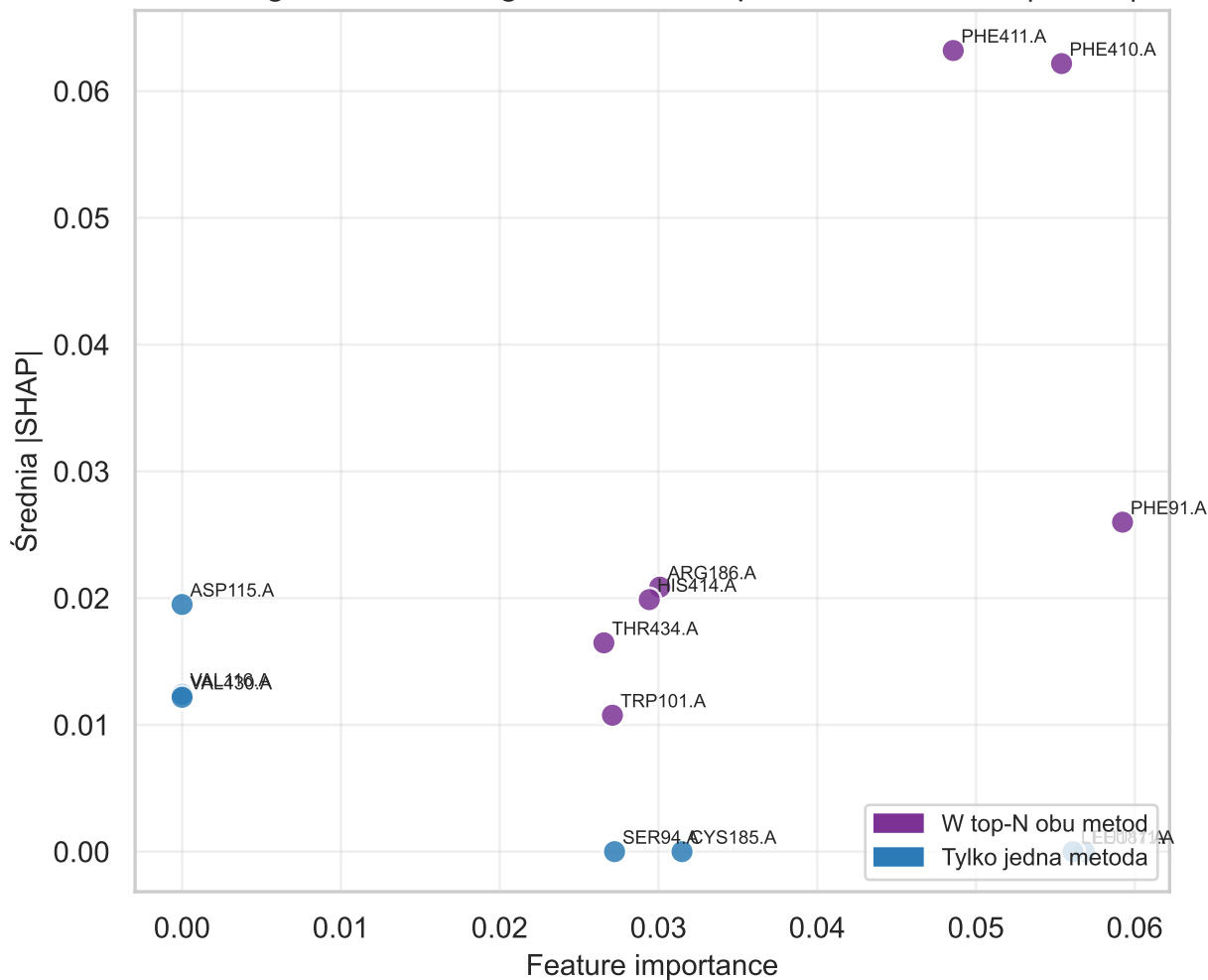
D4 – zgodność rankingów Feature importance i Średnia |SHAP|
