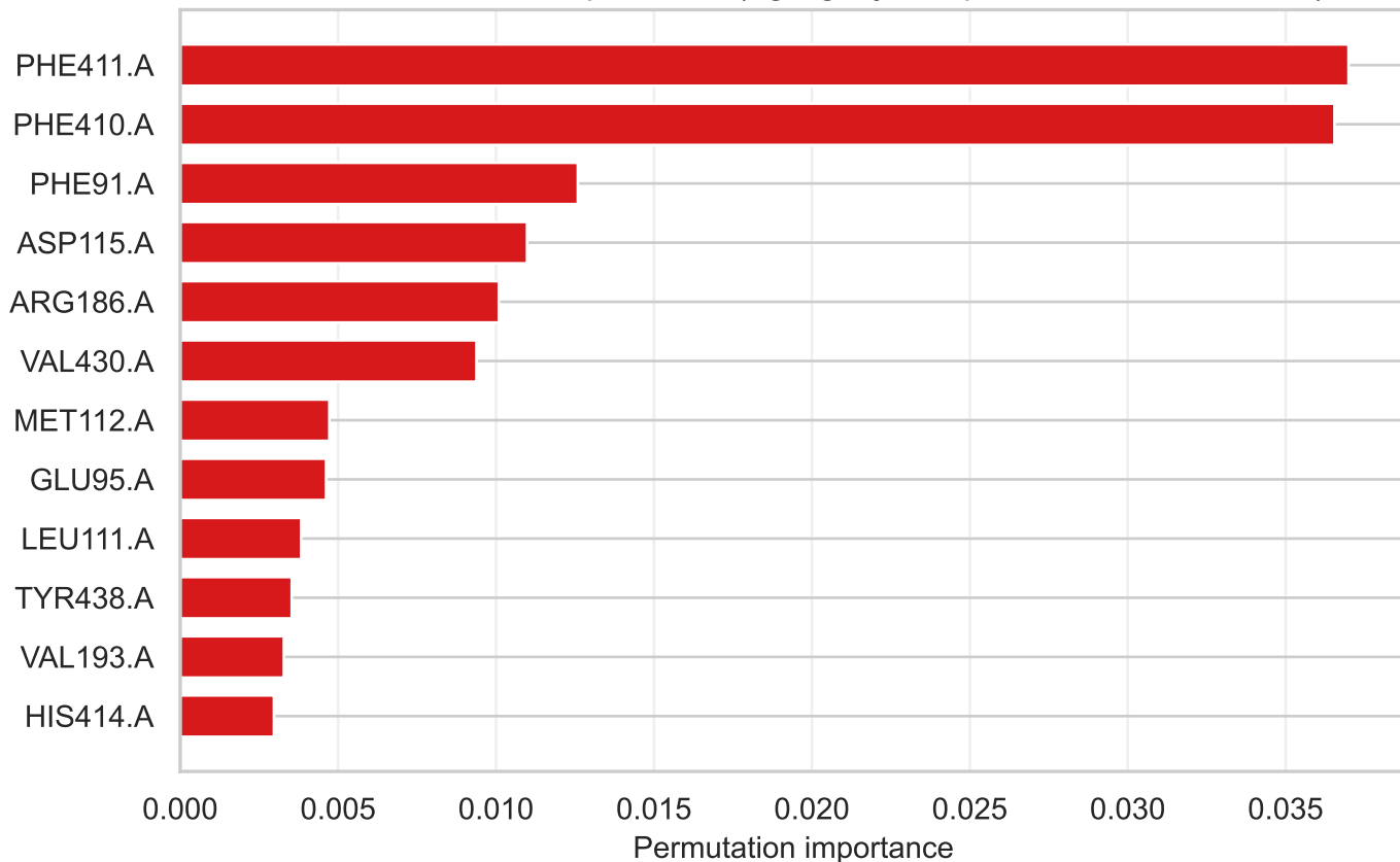
D4 – Permutation importance (agregacja na poziomie aminokwasu)
