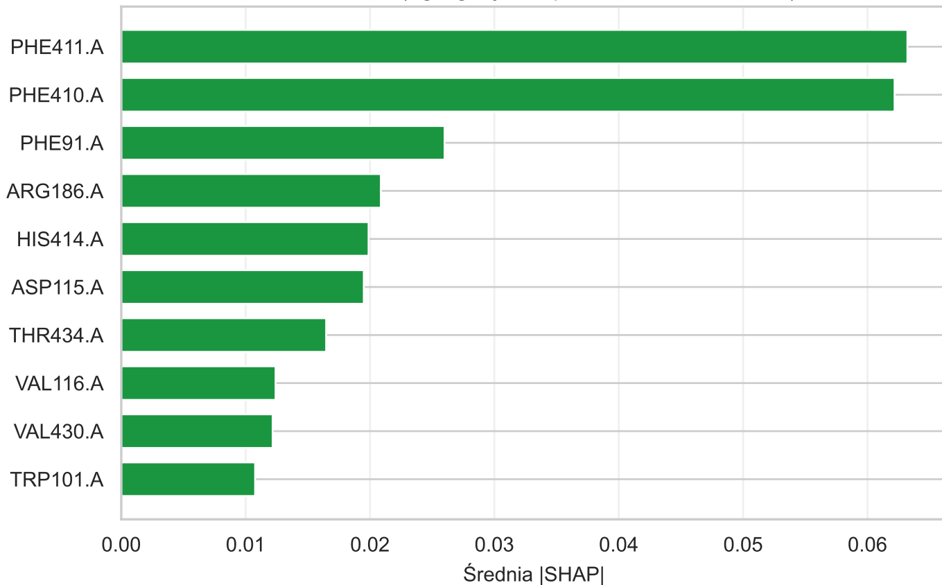
D4 – SHAP (agregacja na poziomie aminokwasu)
