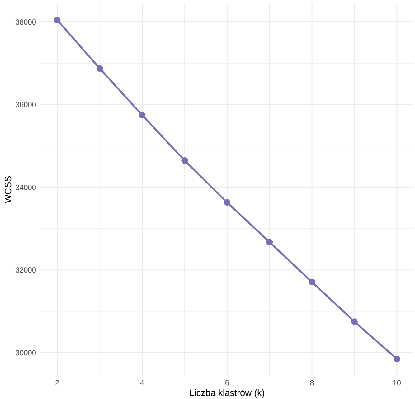
Metoda lokcia (TF-IDF)
