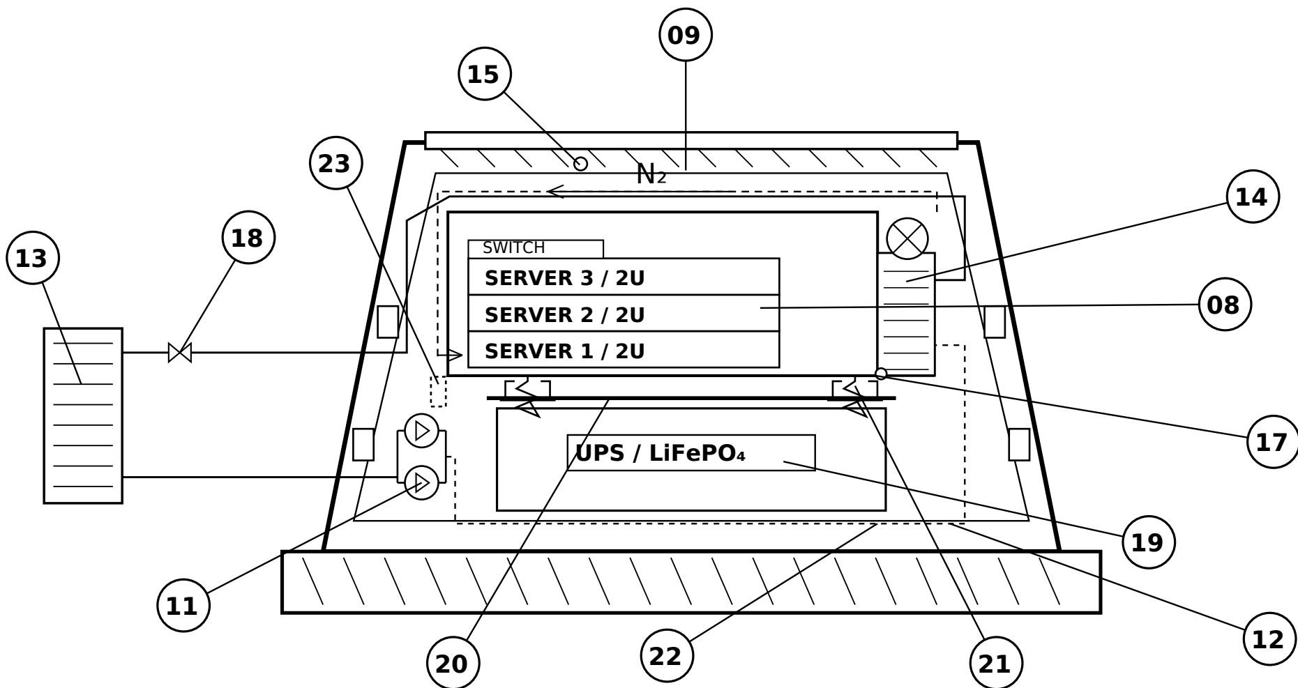
Pompa di dalam wadah; proyeksi digeser agar terbaca.
