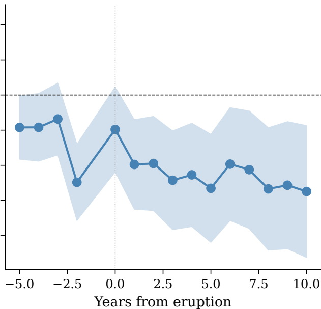
Tambora (1815)
