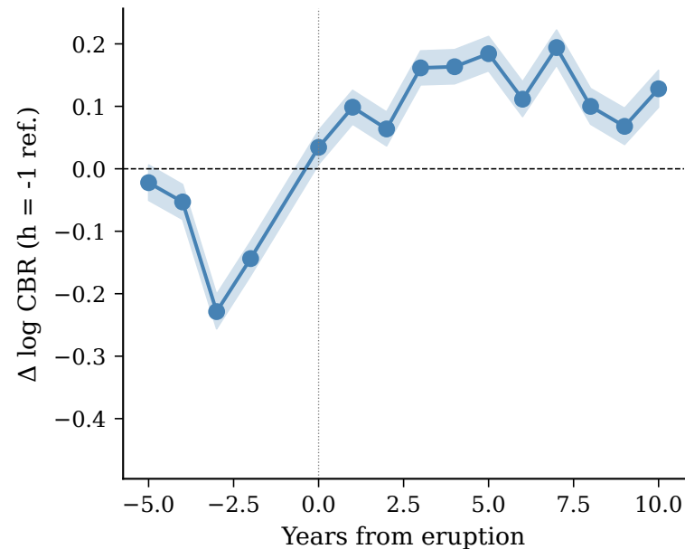
Huaynaputina (1600)
