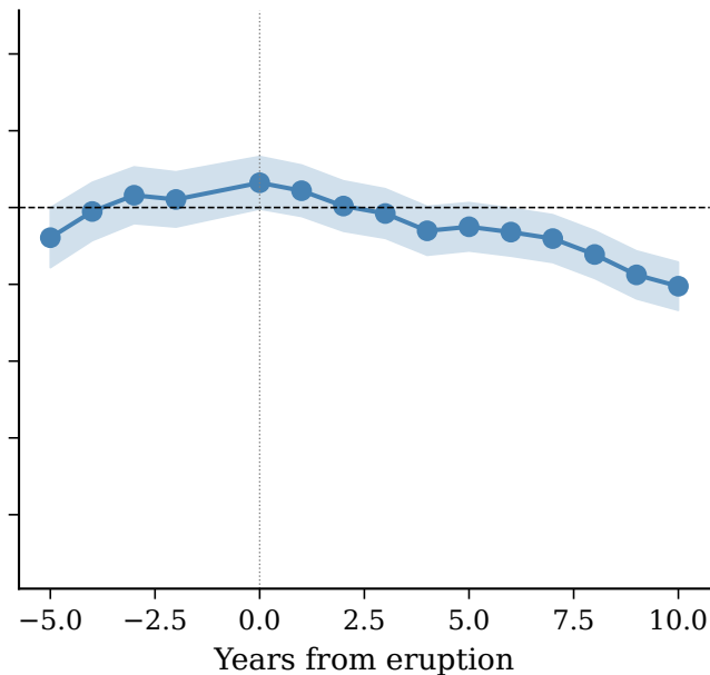
Pinatubo (1991)
