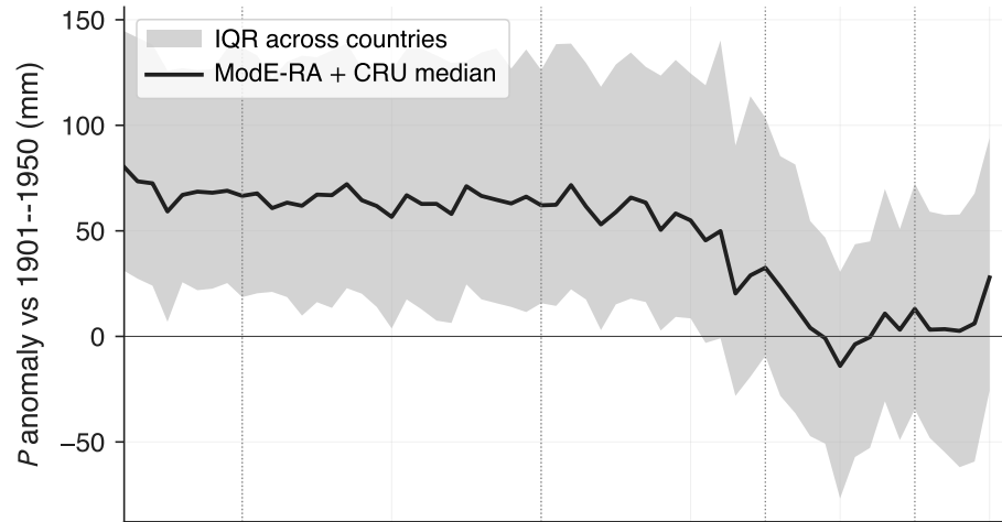
(d) Precipitation uncertainty by decade
