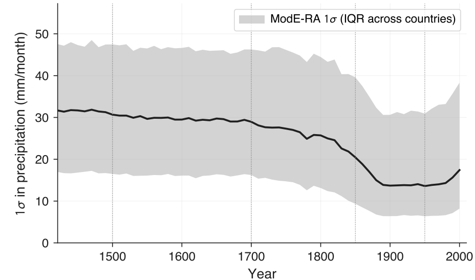
(d) Precipitation uncertainty by decade
