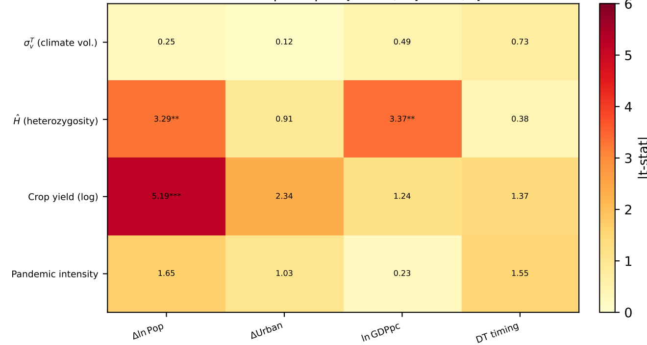
(d) WY-corrected |t-stat| (**p<0.01, **p<0.05, *p<0.10)
