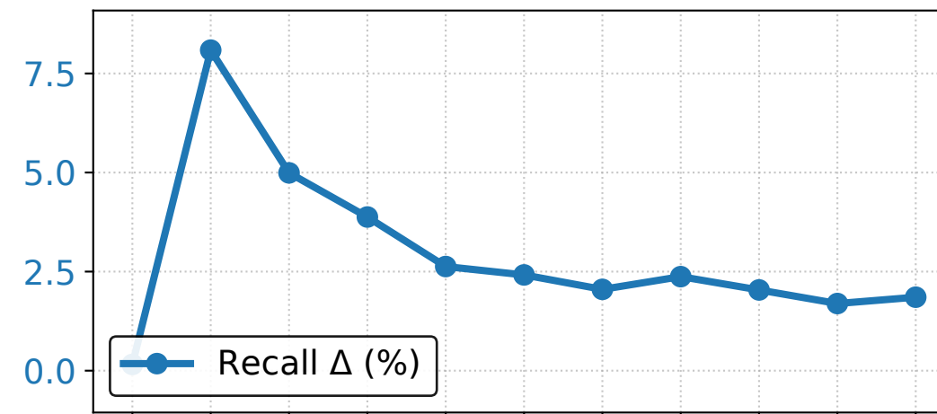
DBpedia
