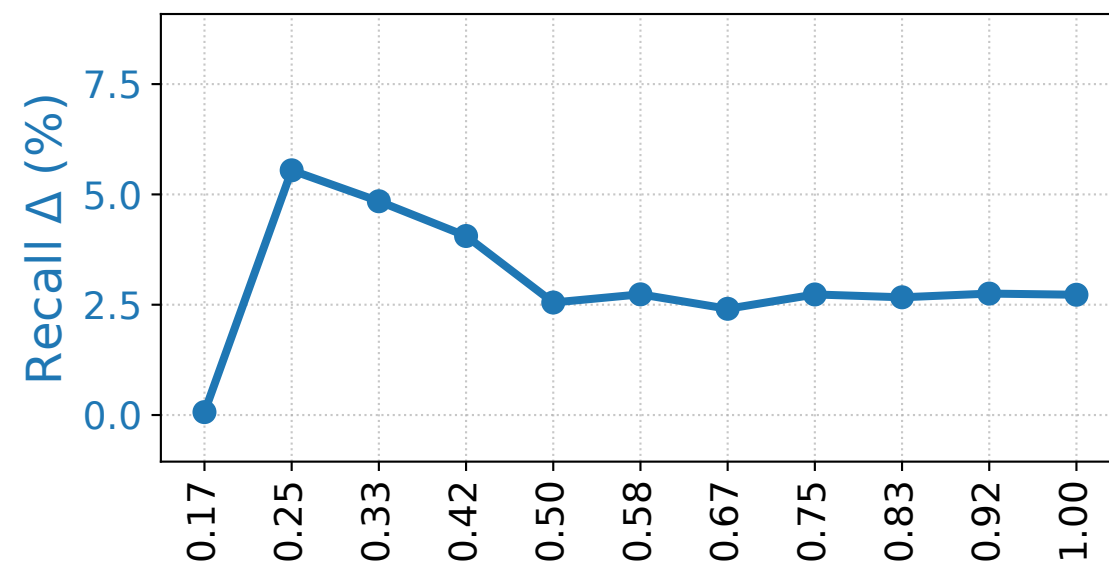
FiQA
