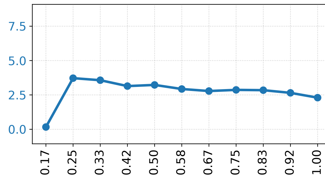
SciDocs
