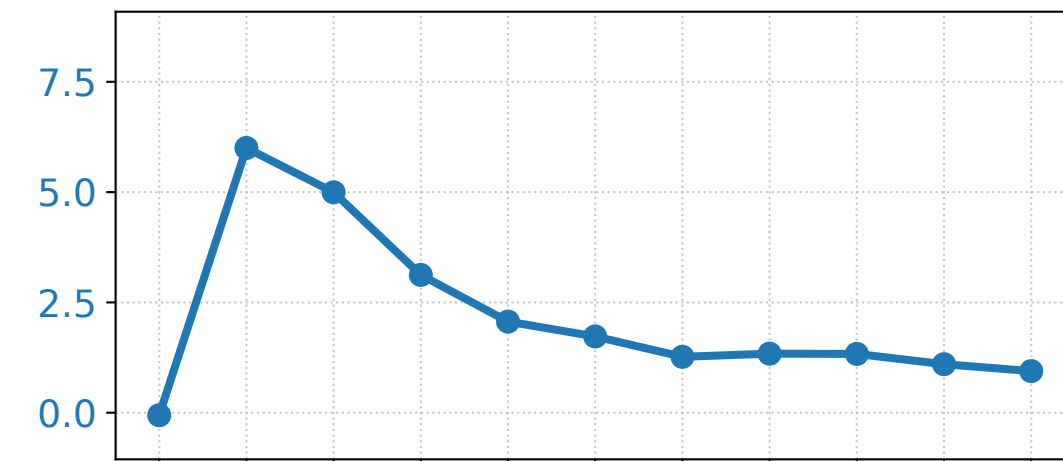
Quora
