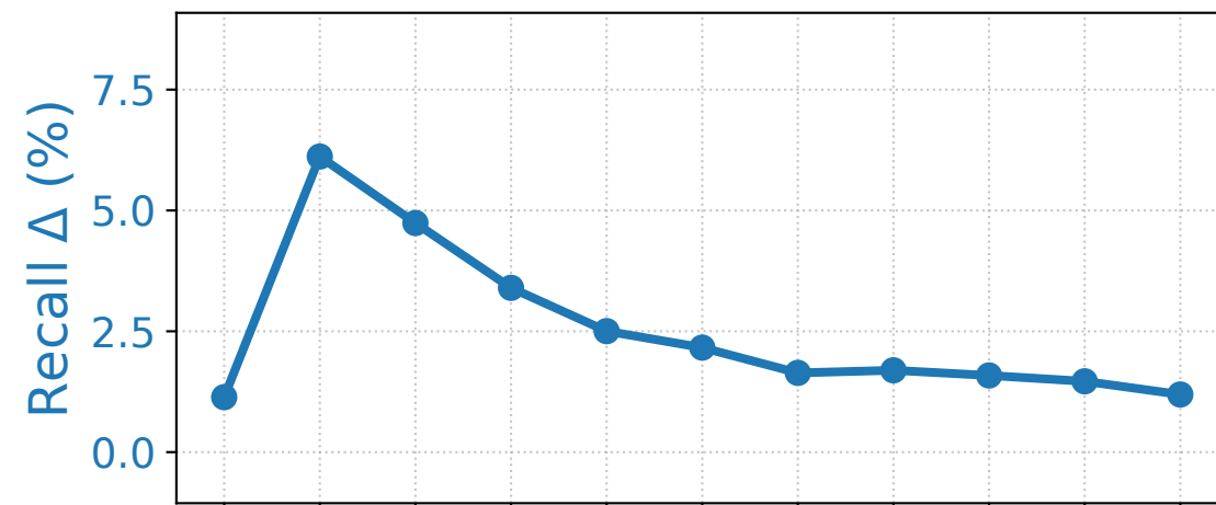
MS Marco
