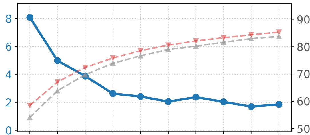
DBpedia
