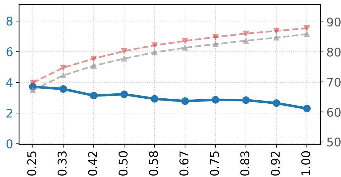
SciDocs
