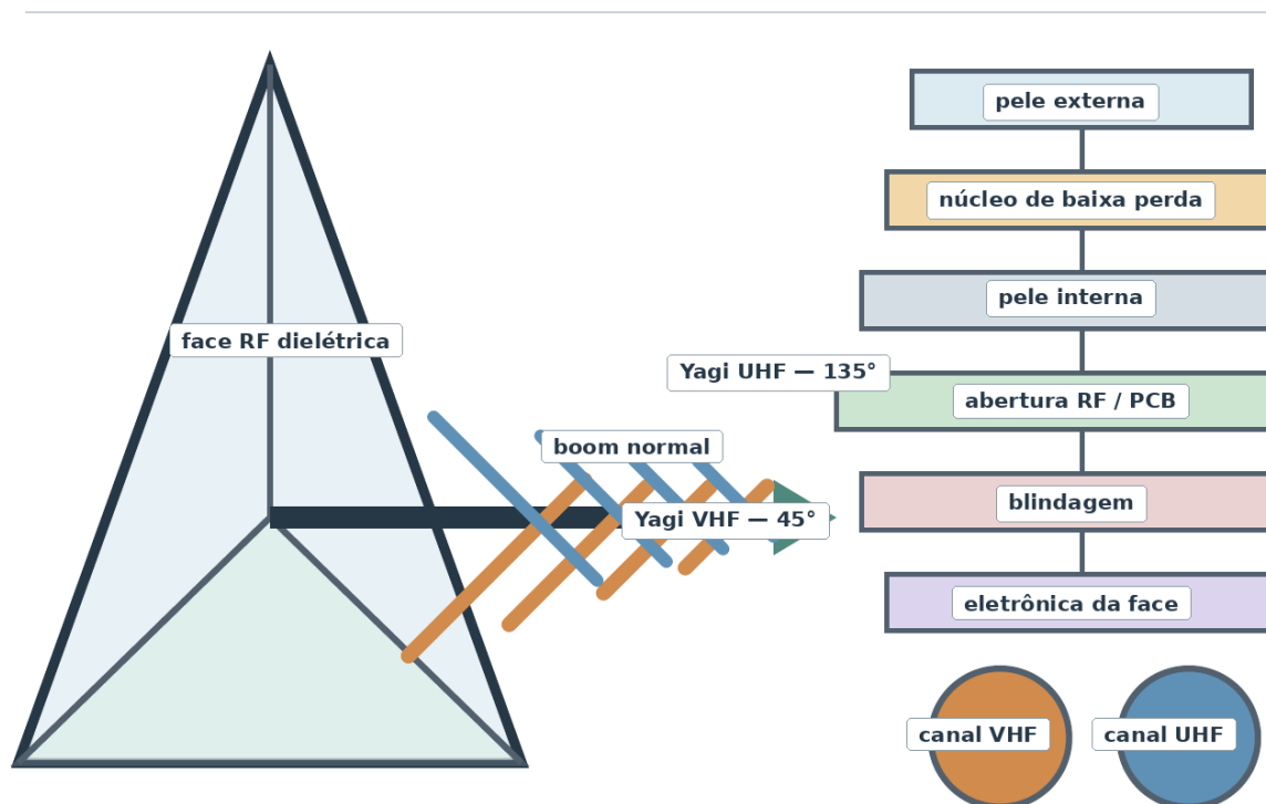
Figura 3 – Montagem de face. O boom escuro segue a normal externa desde o ápice interno e atravessa o centro da abertura triangular de dois metros; os elementos laranja e azul são mutuamente ortogonais e girados conjuntamente em 45° ao redor dessa normal. As placas coloridas à direita representam a pilha de materiais e eletrônica.
