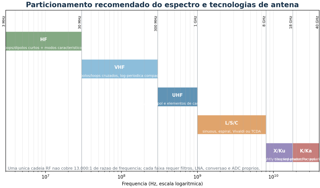
Figure 4.2: Particionamento recomendado do espectro. A escala logarítmica evidencia a incompatibilidade de uma cadeia única.
