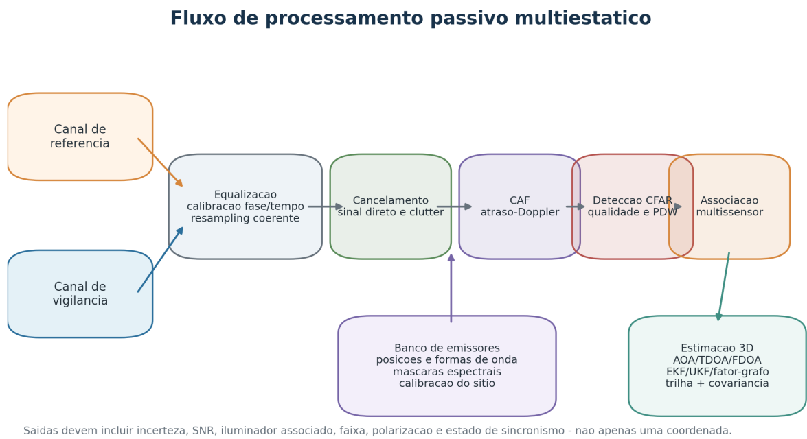
Figure 7.2: Fluxo de referência e vigilância até uma trilha tridimensional com covariância.
