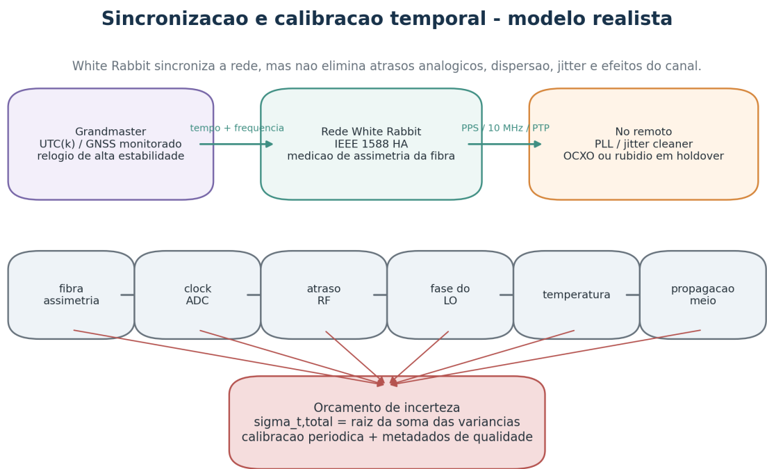
Figure 6.1: Timing and uncertainty budget / Sincronização e orçamento de incerteza.
