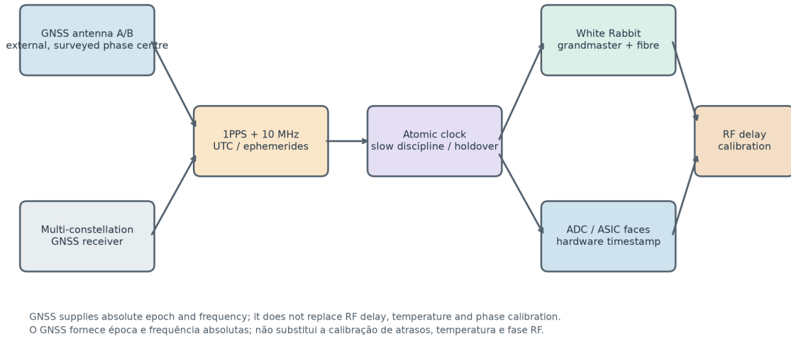
Figure 6.1: Timing and uncertainty budget / Sincronização e orçamento de incerteza.
