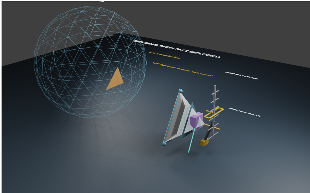
Figure 3.4: Blender 3D model: the VHF Yagi boom is tangent to the face and the support mast is normal to the face / Modelo Blender 3D: a lança da Yagi VHF é tangente à face e a haste de suporte é normal à face.
