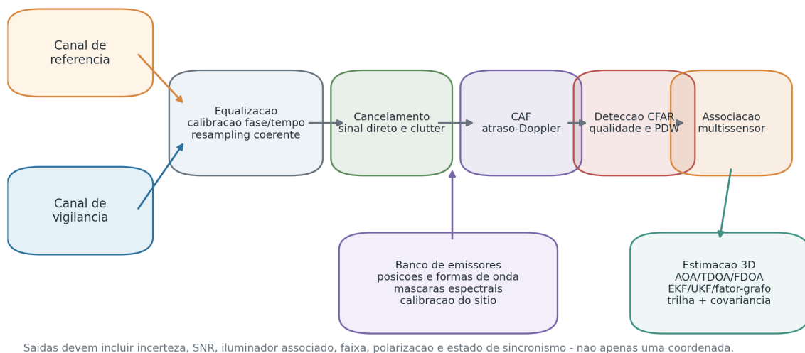
Figure 7.2: Multistatic passive processing / Processamento passivo multiestático.
