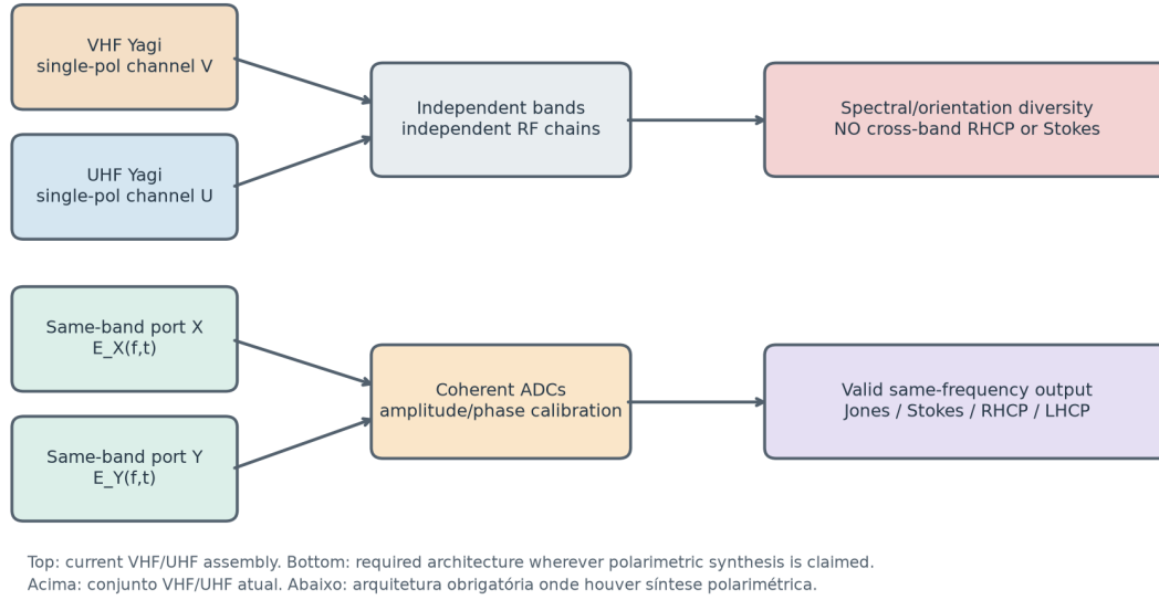
Figure 4.2: Cross-band diversity versus valid same-band polarimetric acquisition / Diversidade entre faixas versus aquisição polarimétrica válida na mesma faixa.
